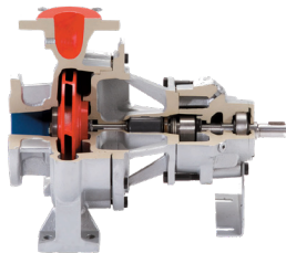
Centrifugal
