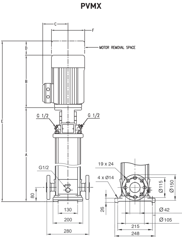
ANSI 250# Flanges
