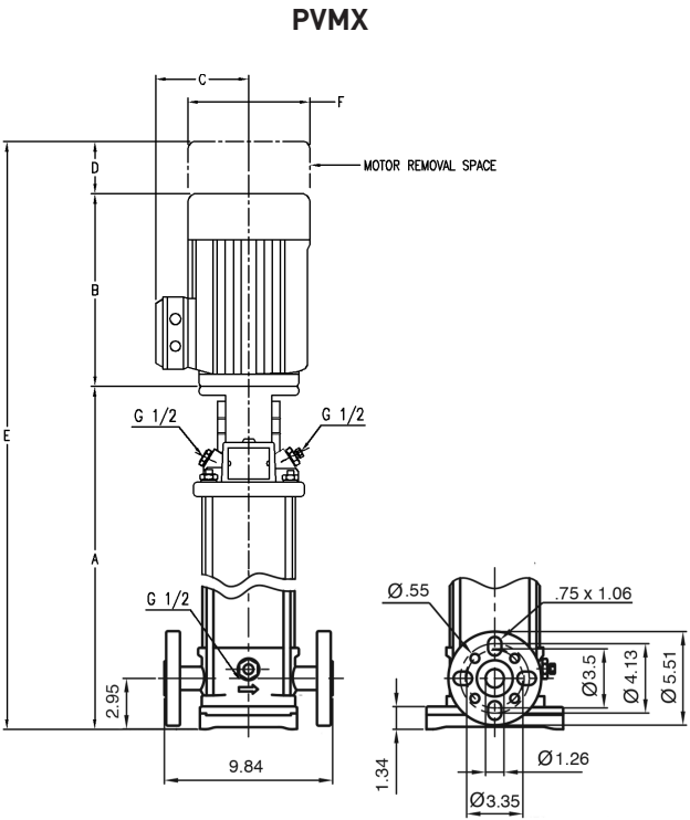
ANSI 250# Flanges
