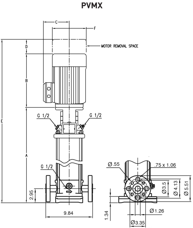
ANSI 250# Flanges
