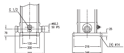
ANSI 250# Flanges
