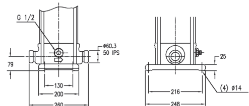
ANSI 250# Flanges
