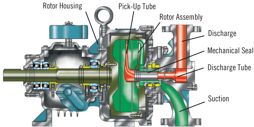
Roto-Jet API-R11
